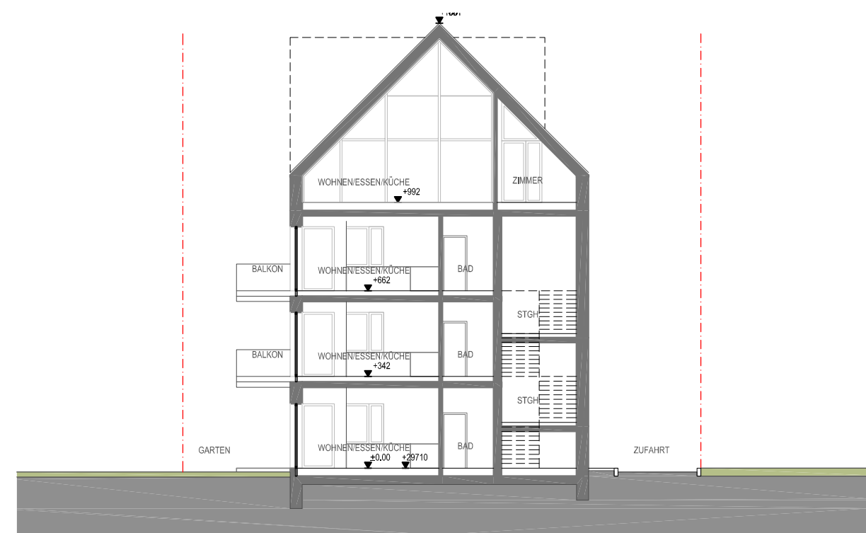
SCHNITTE
