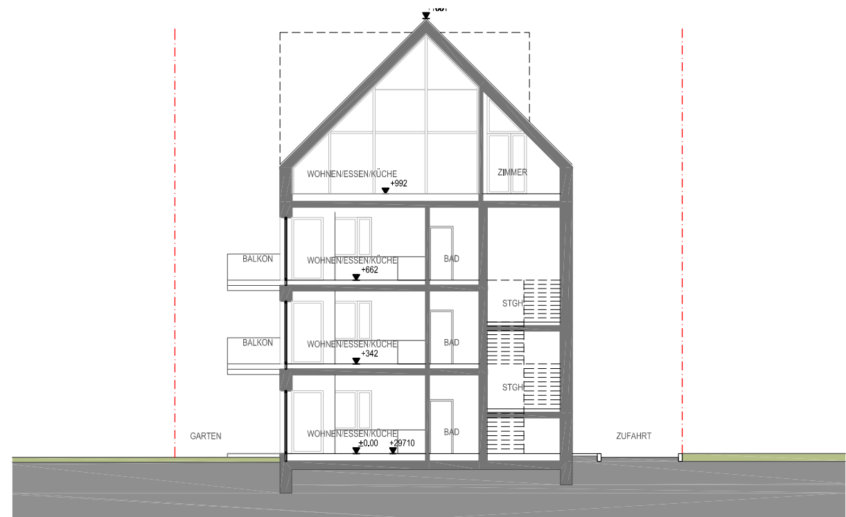
SCHNITTE
